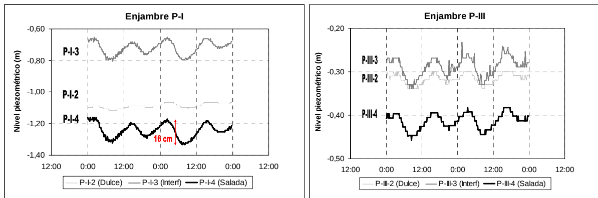
Fig. 6. Fluctuación de niveles piezométricos (m.s.n.m.) durante 48 horas en estado natural (10 y 11 de junio de 2006) en P-I y P-III.
