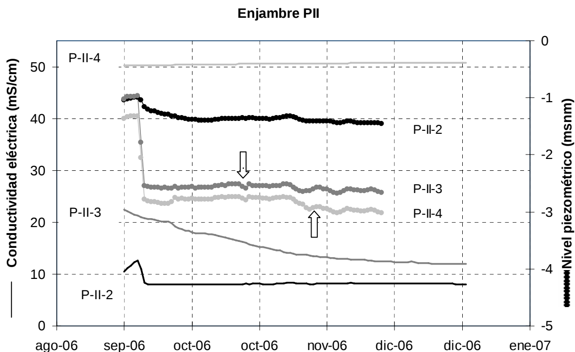
Figura 7. Evolución de nivel piezométrico y conductividad eléctrica de los piezómetros puntuales del enjambre P-II.
