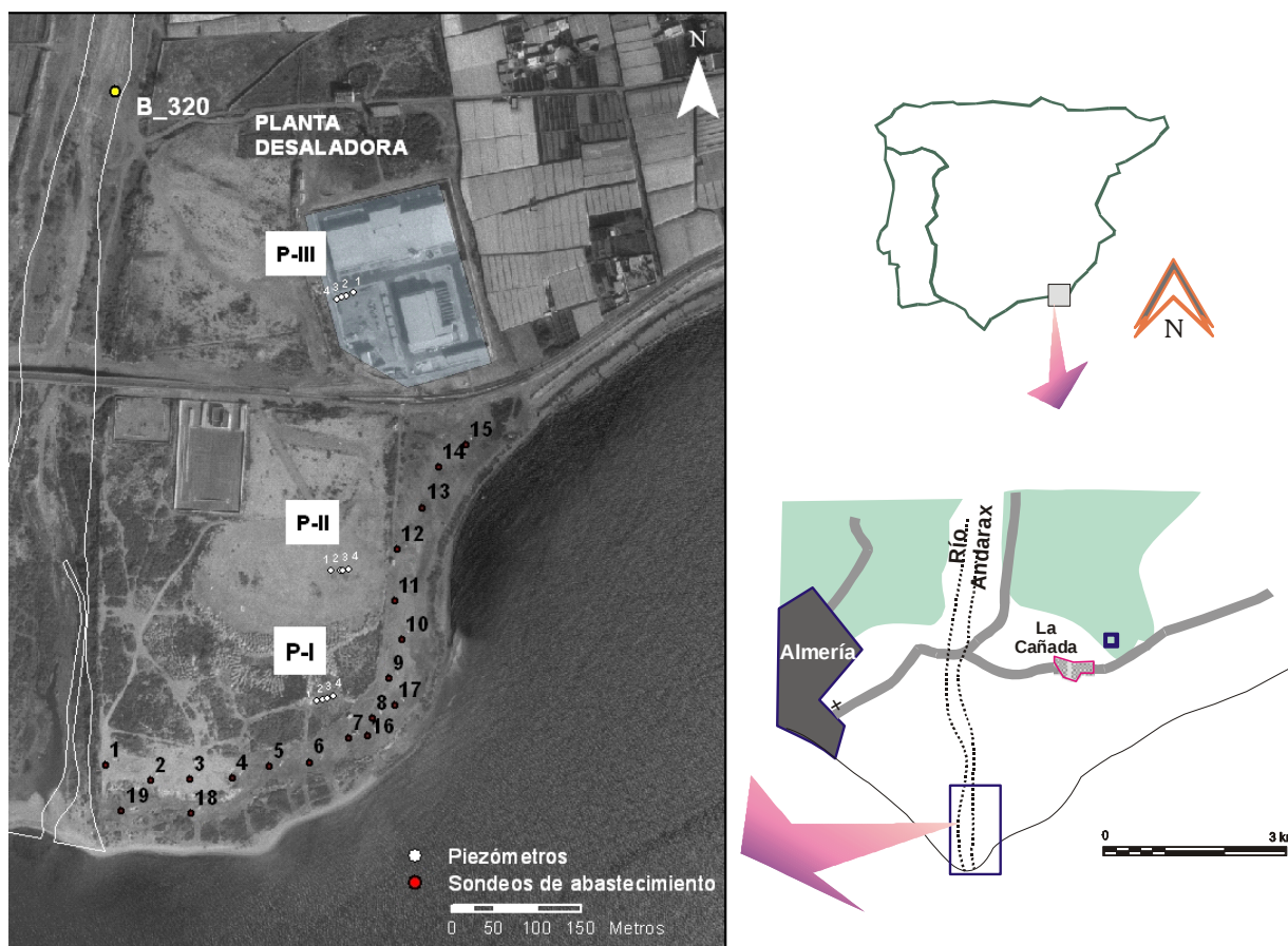
Figura 1. Situación de de la planta desaladora de agua de mar de Almería, indicando los sondeos de captación y los tres grupos de piezómetros de control (P-I, P-II y P-III).
