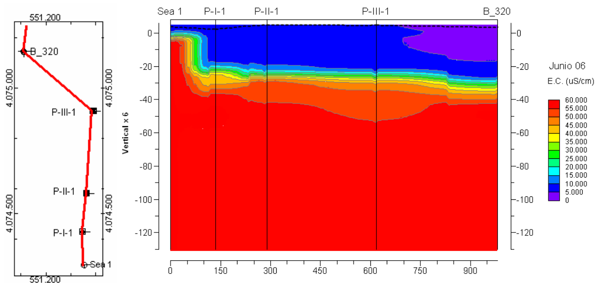
Figura 4. Perfil de conductividad eléctrica en el delta del Andarax en estado natural, junio de 2006, sin bombeos por parte de la planta desaladora. En el cuadro de la izquierda se representa en planta los piezómetros utilizados para el perfil.
