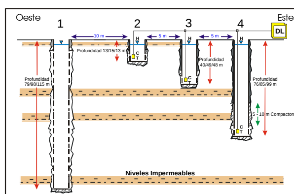
b) esquema de los enjambres de piezómetros y los sensores de medida en continuo.
