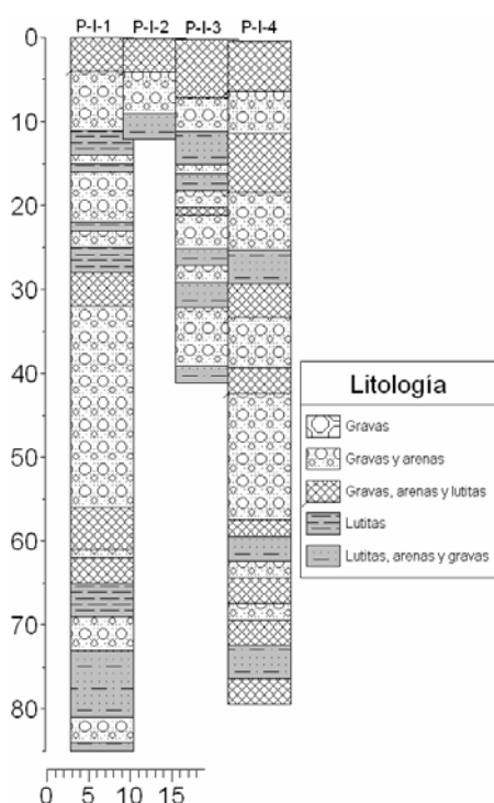
Figura 2. Litología del grupo de piezómetros P-I.
