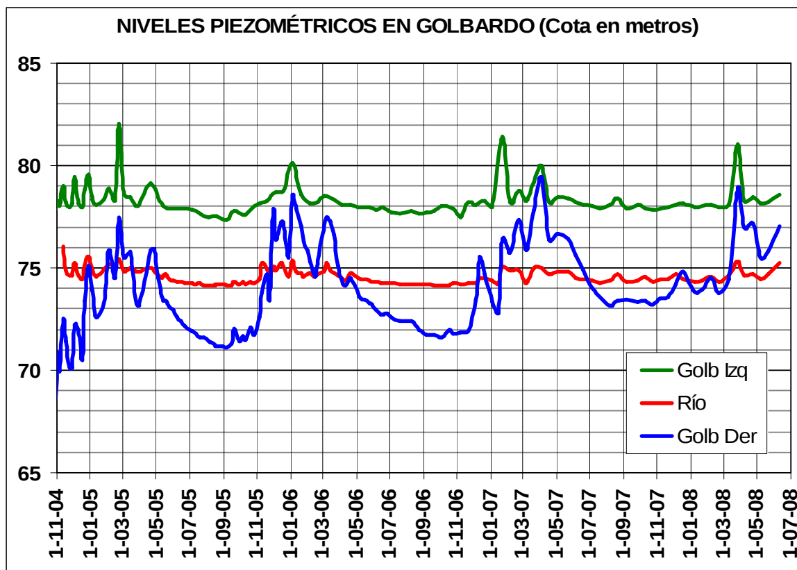
Figura 7. Piezometría en el oeste (Golbardo / Barcenaciones)
