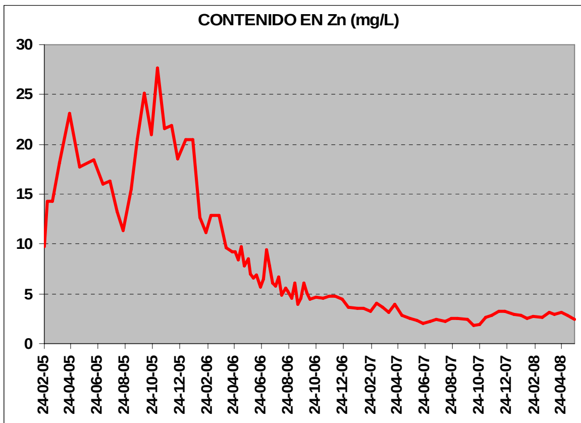
Figura 11. Agua de inundación. Contenido en zinc
