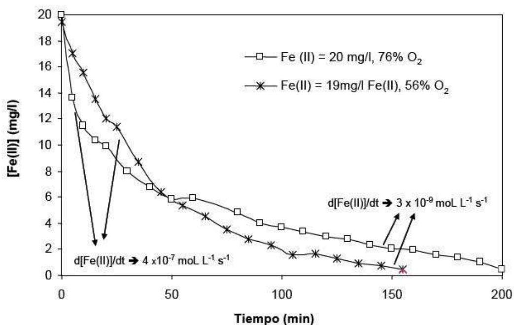
Figura 13. Experimento de oxidación de Fe(II) en agua equilibrada con dolomía de Reocin. Condiciones de Fe(II)=20mg/L y déficit de oxígeno disuelto (E. López Pamo, J. Sánchez España " et al ". IGME)
