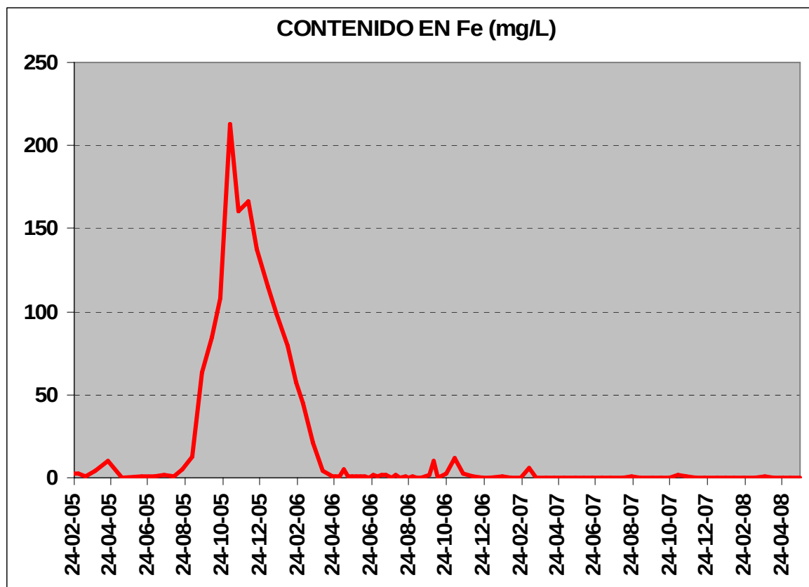
Figura 10. Agua de inundación. Contenido en hierro
