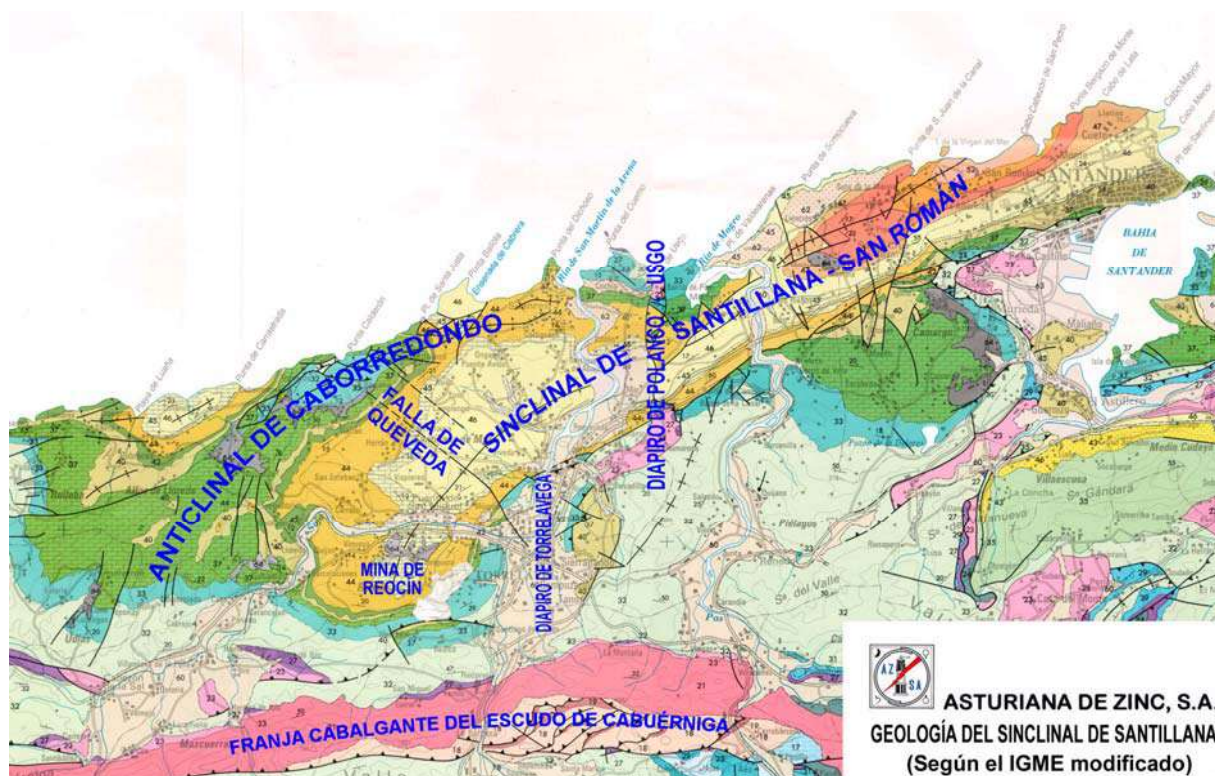
Figura 2. Mapa geológico
