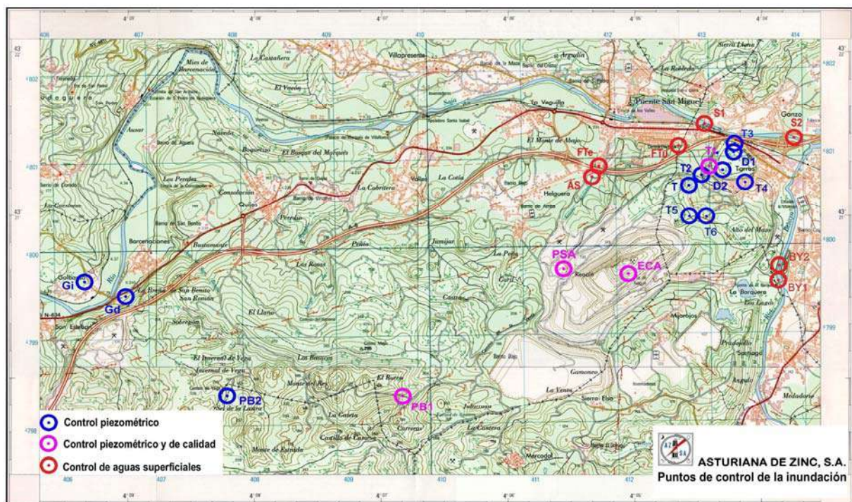
Figura 4. Plan de actuación medioambiental. Puntos de control
