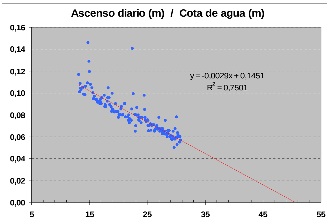
Figura 6. Ascenso diario frente a cota del agua
