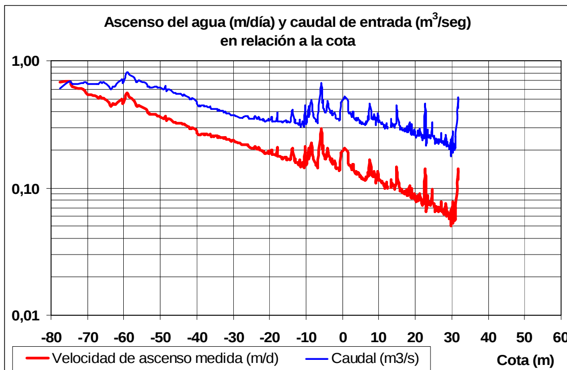
Figura 5. Velocidad de ascenso del agua en metros por día y caudal de entrada en metros cúbicos por segundo, en relación con la cota del agua
