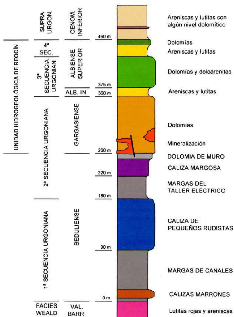
Figura 3. Columna estratigráfica
